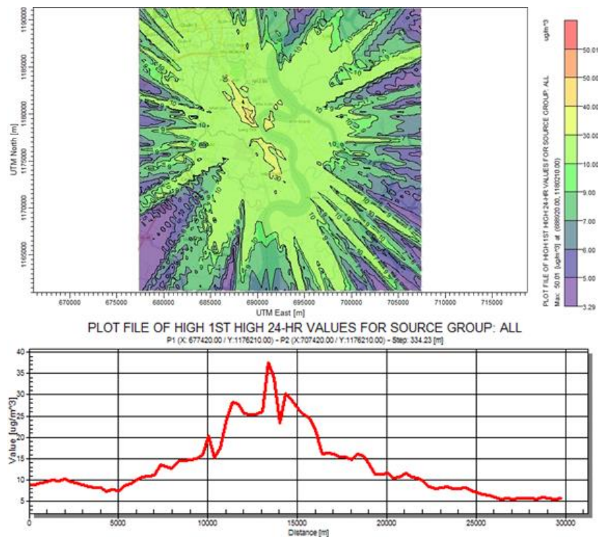
(e) TSP trung bình 24 giờ mô hình ISCST3
