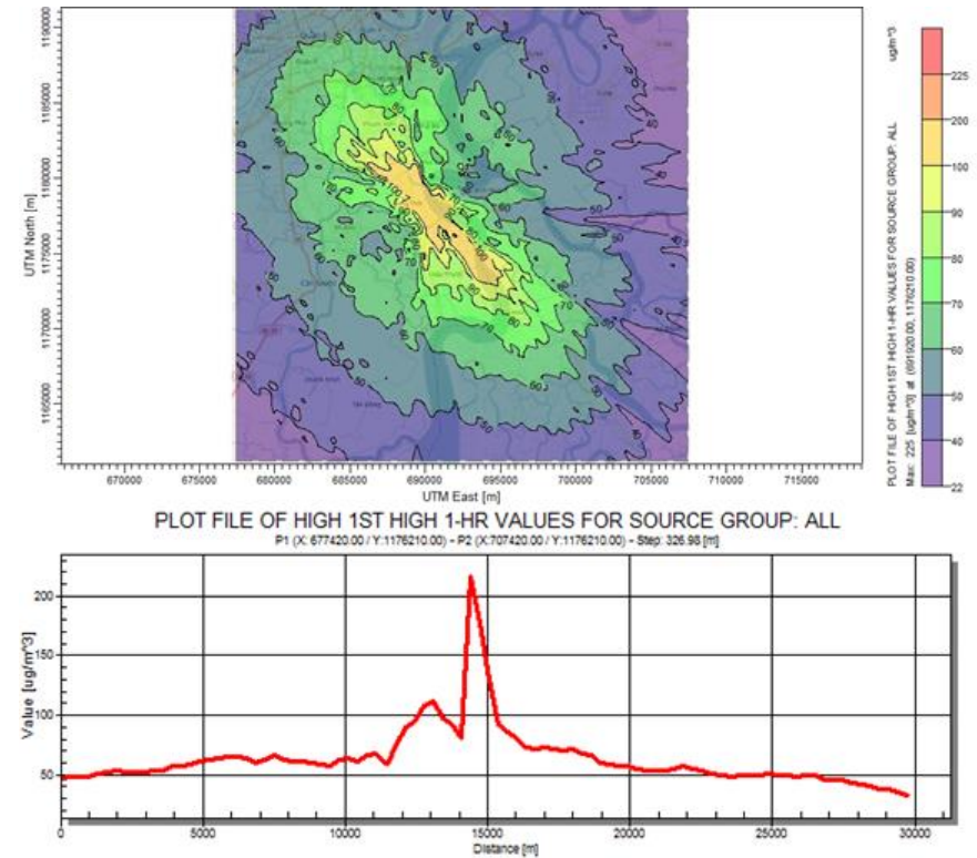
(f) TSP trung bình 1 giờ mô hình AERMOD
