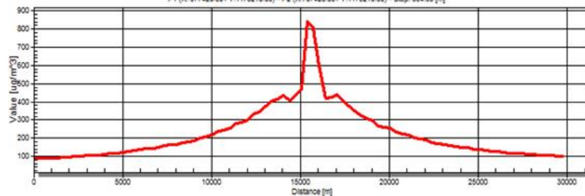
(b) \text{SO}_2 trung bình 1 giờ mô hình AERMOD
