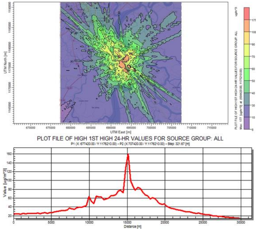
(c) SO 2 trung bình 24 giờ mô hình ISCST3
