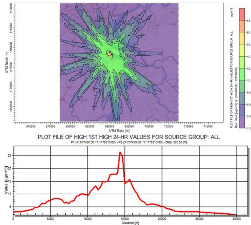
(f) TSP trung bình 24 giờ mô hình AERMOD
