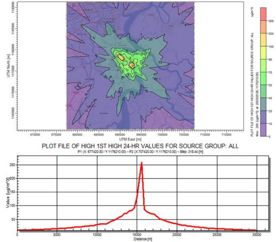
(d) SO 2 trung bình 24 giờ mô hình AERMOD
