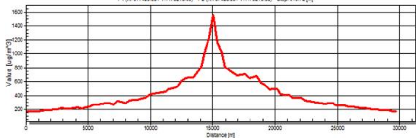
(a) \text{SO}_2 trung bình 1 giờ mô hình ISCST3
