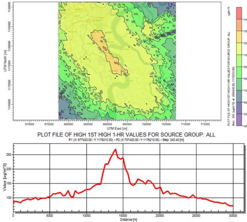
(e) TSP trung bình 1 giờ mô hình ISCST3
